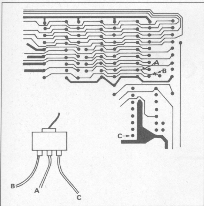
Figura 3 - Placa de CI (face inferior)
